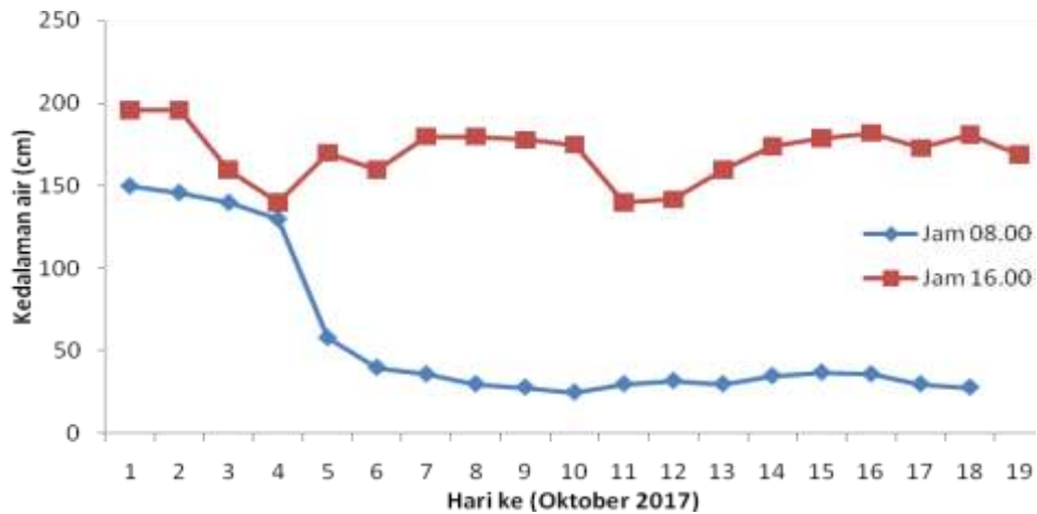
Gambar 3.3. Dinamika muka air di saluran sekunder pagi dan sore hari pada bulan Oktober 2017
