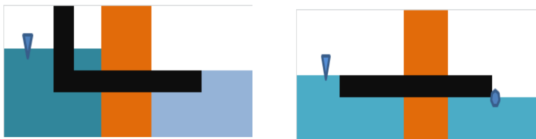
Gambar 2.2. Pintu air leher angsa posisi retensi air (a), pintu dirubah menjadi drainase (b)
