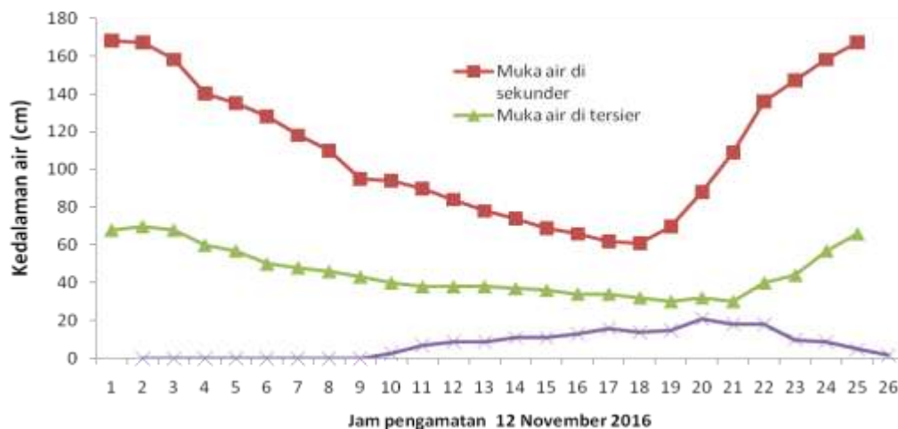
Gambar 3.2. Dinamika muka air tanah dan air di saluran setiap jam pada kondisi musim hujan.
